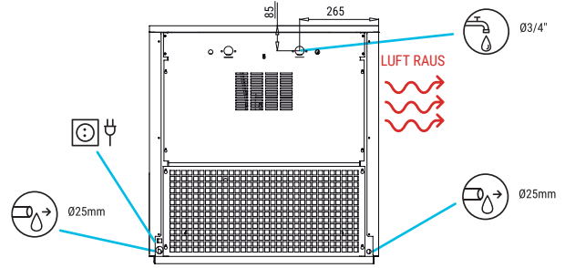
RÜCKANSICHT
