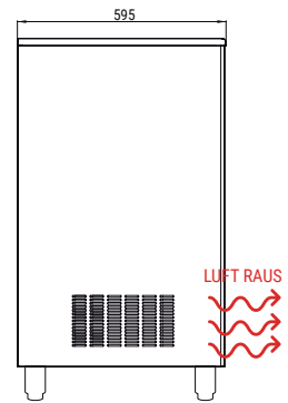
LINKE SEITENANSICHT
