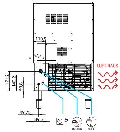
RÜCKANSICHT
