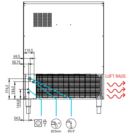
RÜCKANSICHT
